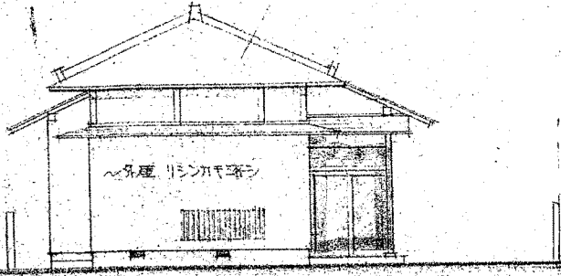
西立面図 1:100
