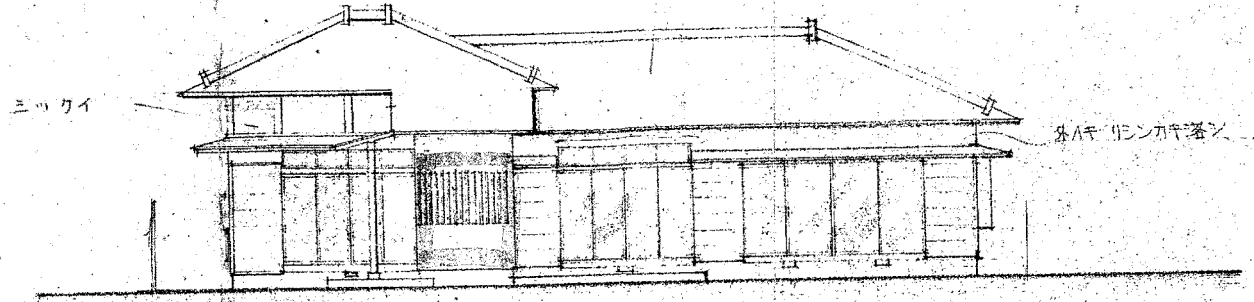
南立面図 1:100
